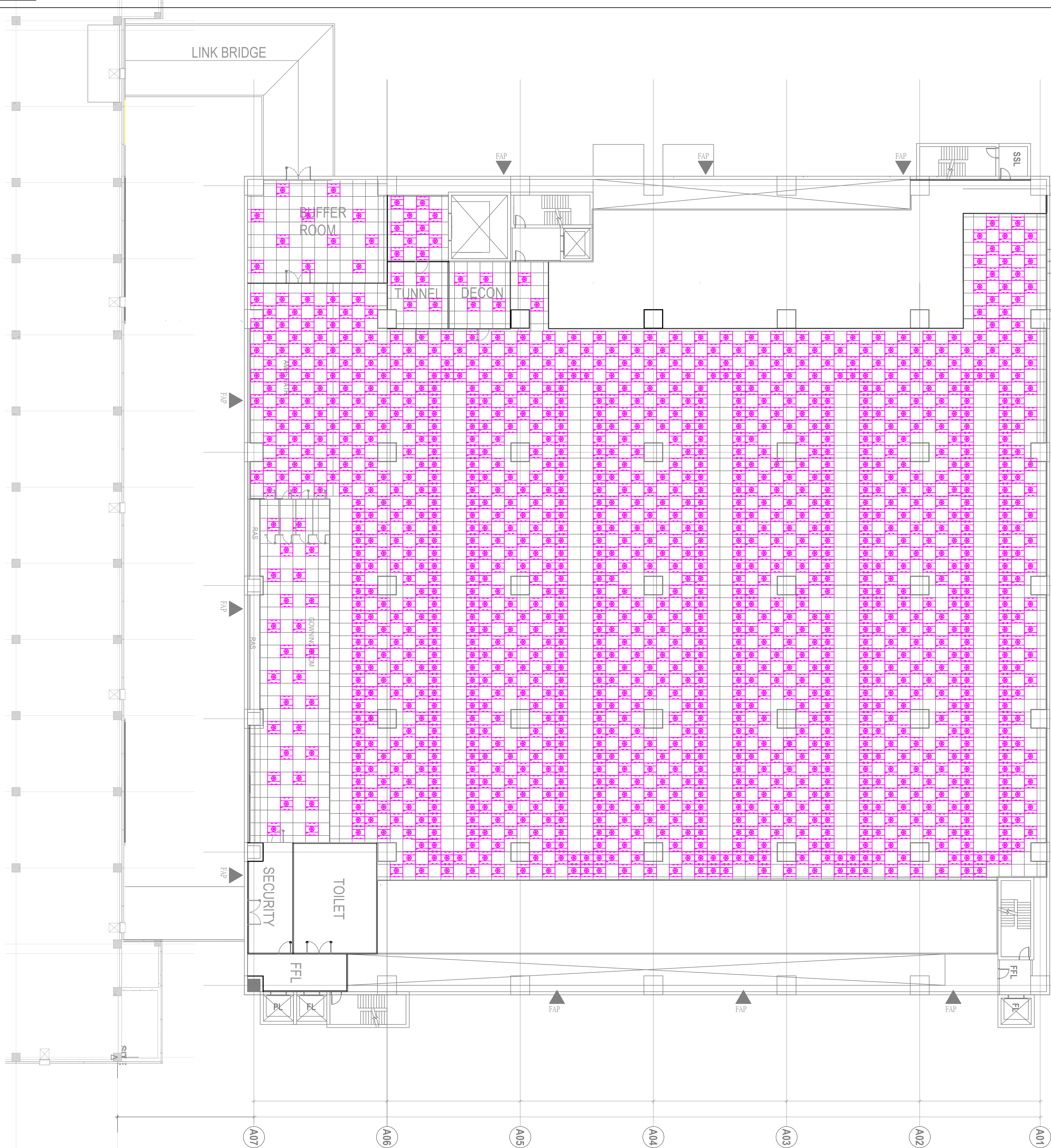
F10E1 L30 FFU LAYOUT SCALE 1:200
